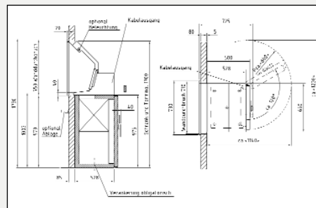
CASHDROP ecco inwall nach Zeichnung A-ELS 200-000-46-3-00
